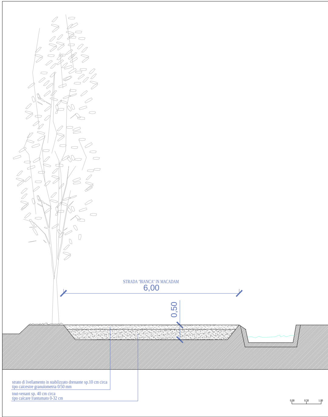
progetto - sezione tipo strada di accesso
